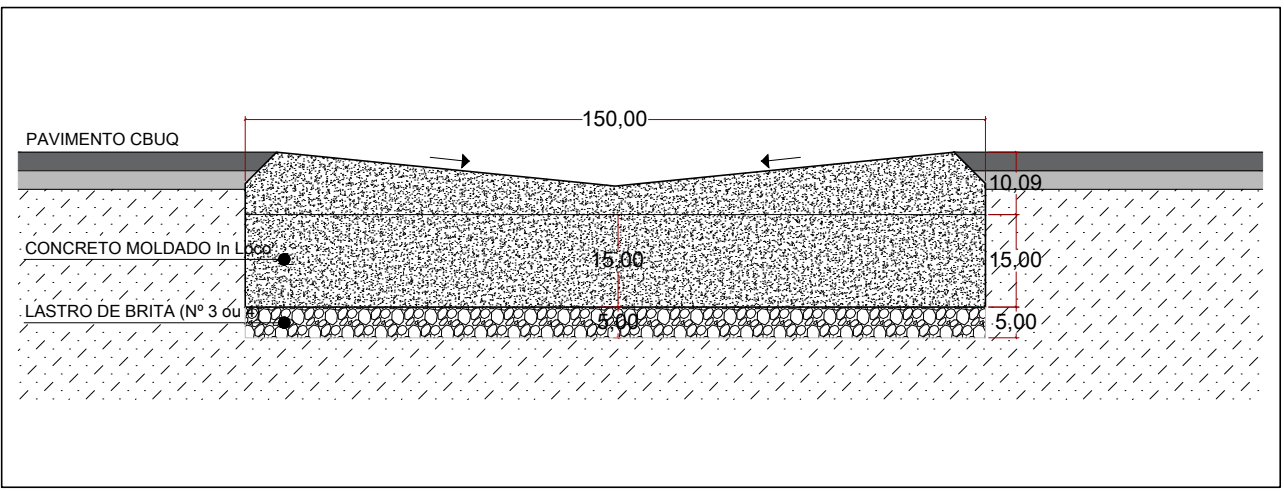
DET. SARJETÃO EM CONCRETO SEM ESCALA
