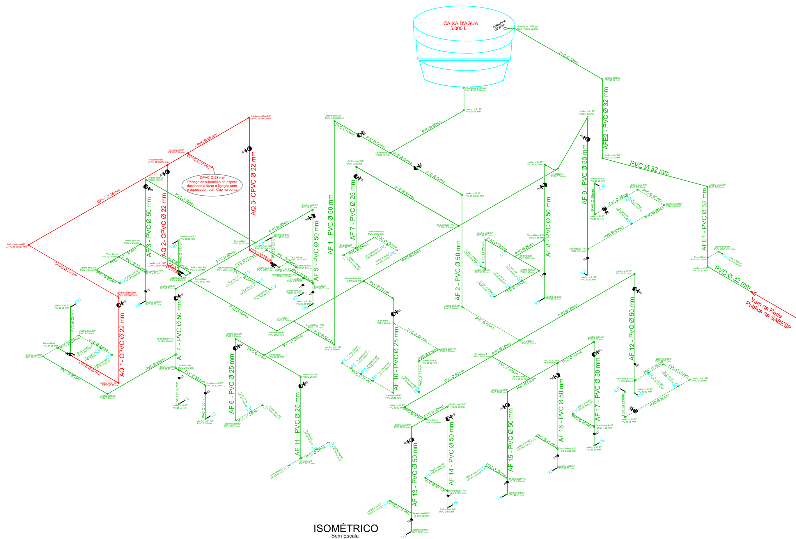
ISOMÉTRICO
