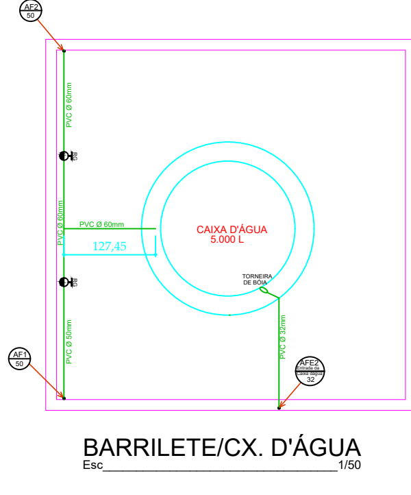
BARRILETE/CX D'ÁGUA
