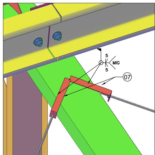
DET-4 s/e
