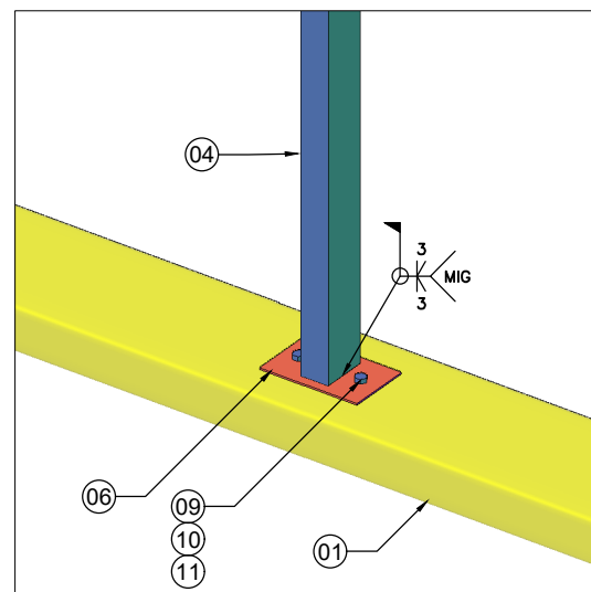
DET-1 s/e
