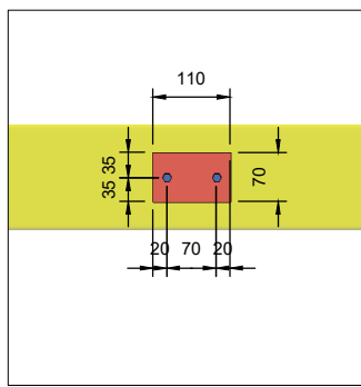
DET-1 s/e
