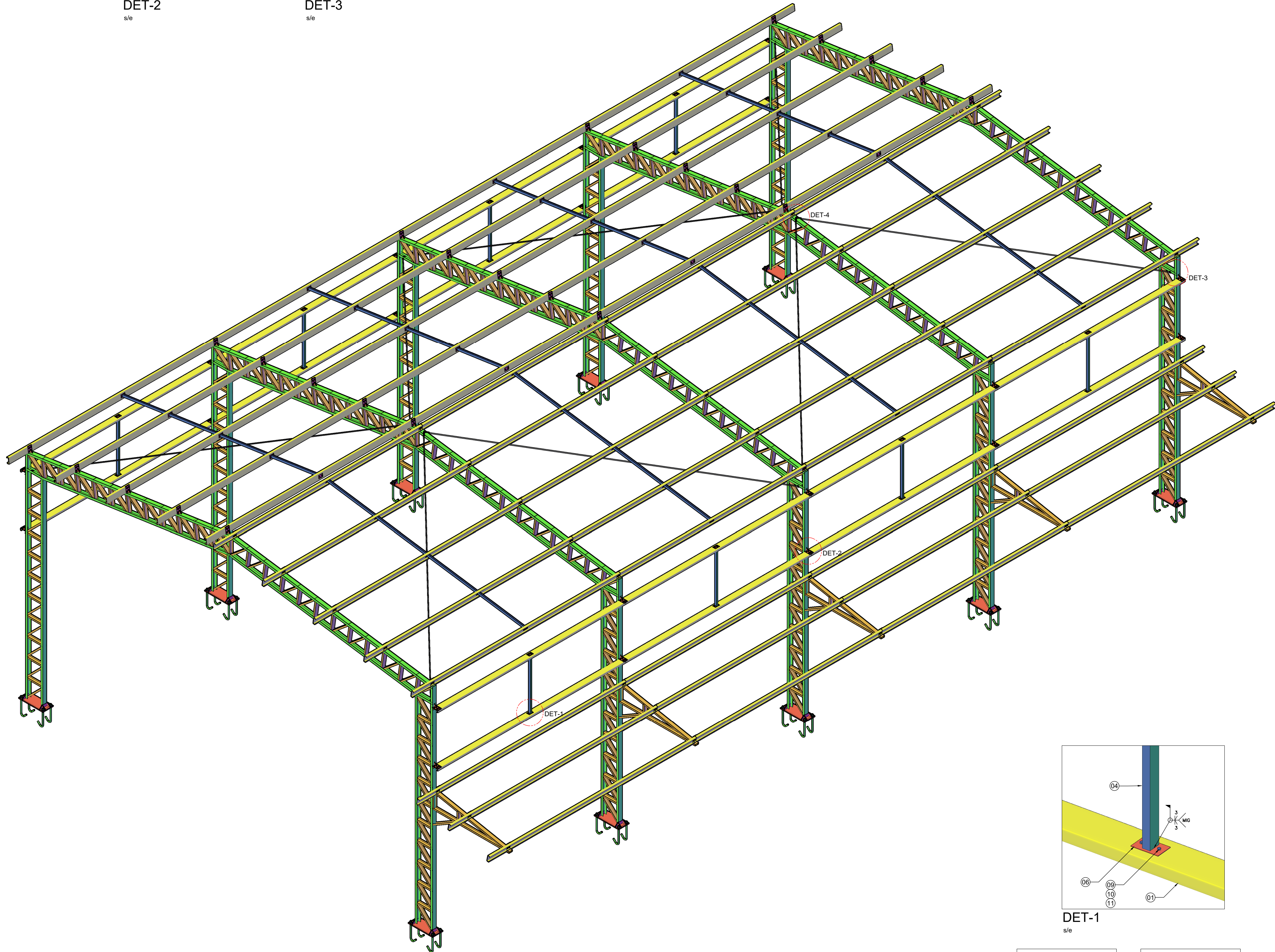
DET-4 s/e
