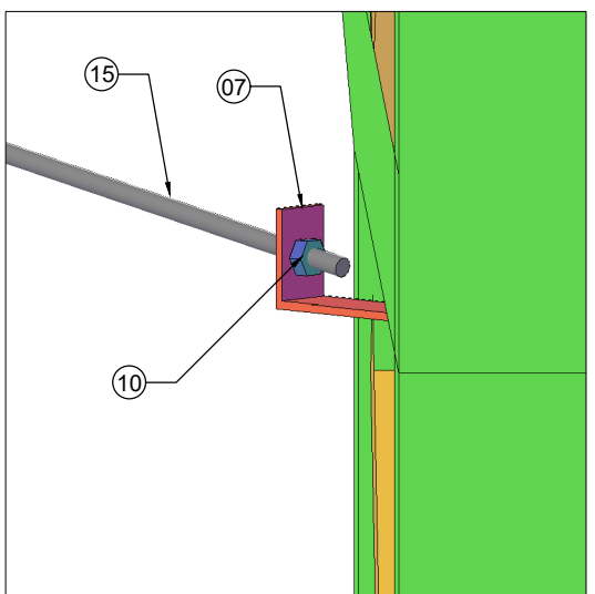
DET-3 s/e
