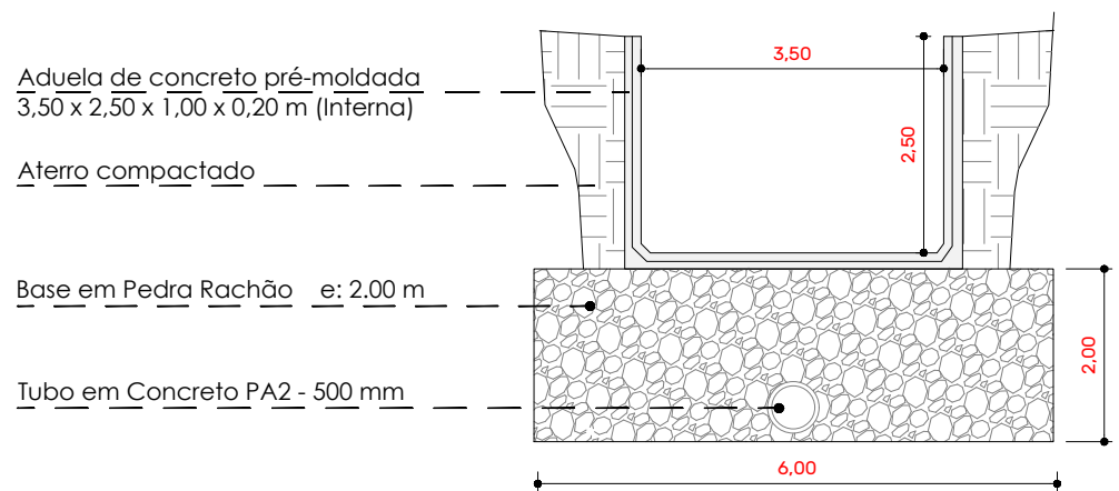
DETALHAMENTO - ADUELA ABERTA
