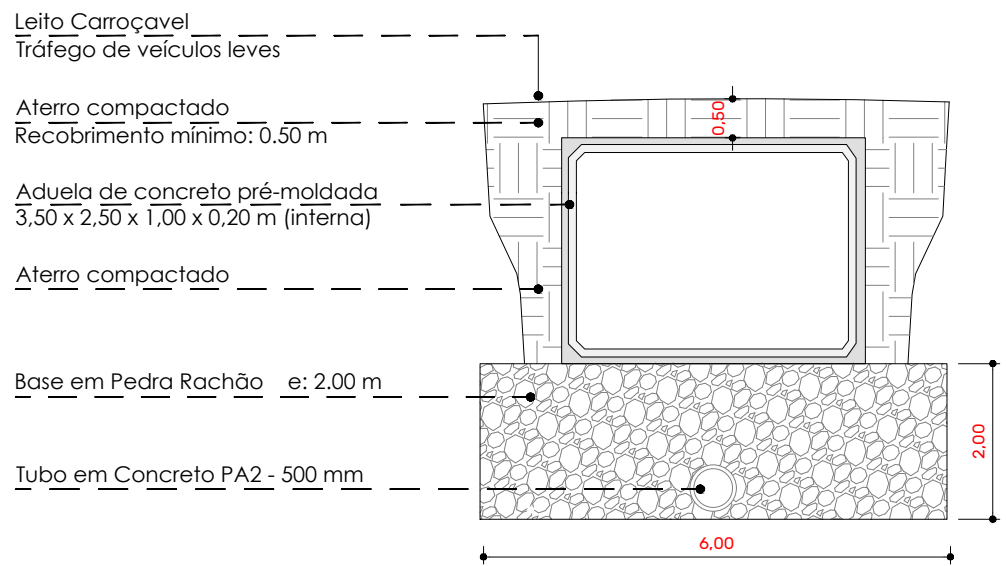
DETALHAMENTO - ADUELA FECHADA
