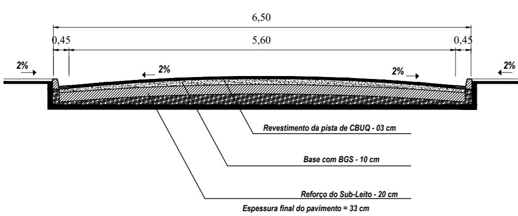
DETALHE GENÉRICO
