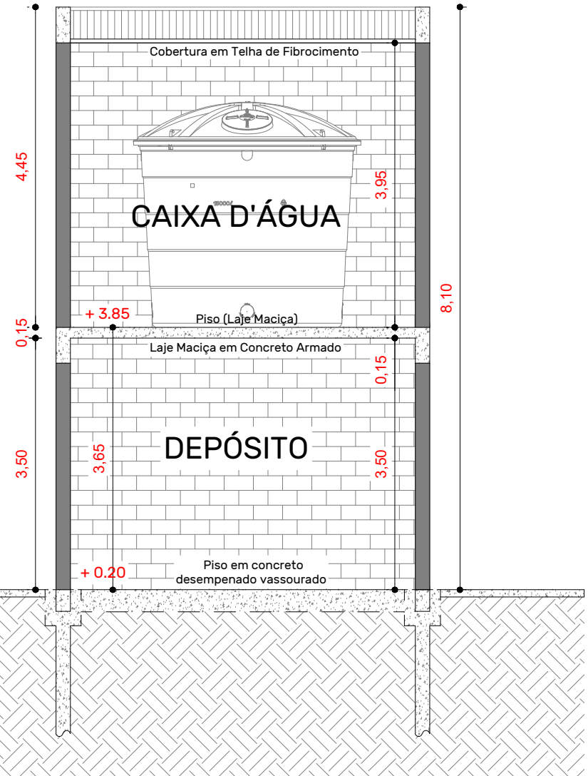
CORTE TRANSVERSAL ESQUEMÁTICO (BB) Esc. 1/75
