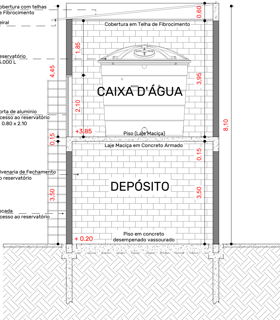
CORTE TRANSVERSAL ESQUEMÁTICO (AA) Esc. 1/75
