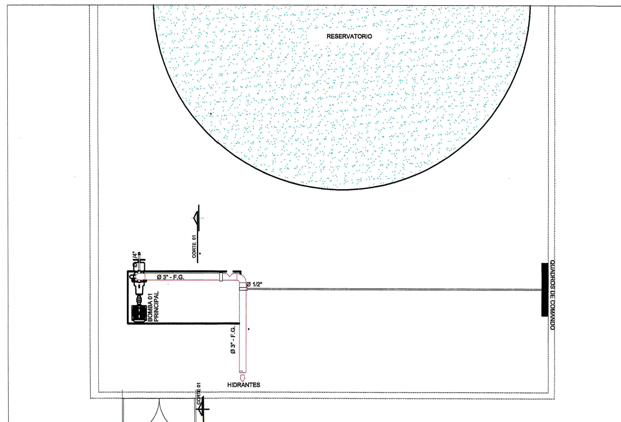
PLANTA BAIXA (NIVEL SUPERIOR) Escala 1:50
