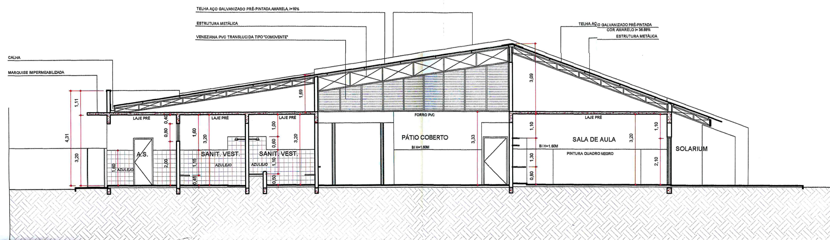
CORTE B-B
