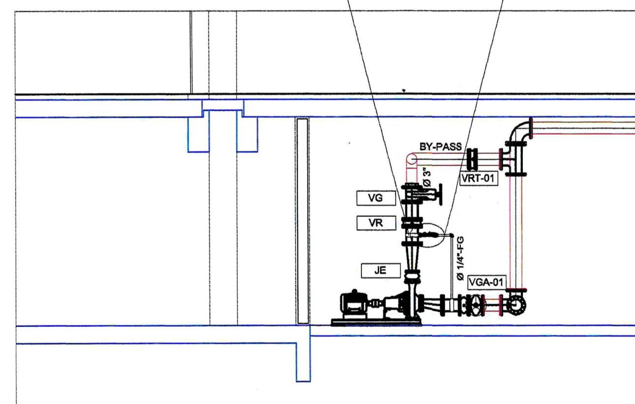
CORTE -01 (SISTEMA REDE DE HIDRANTES) Escala 1:50
