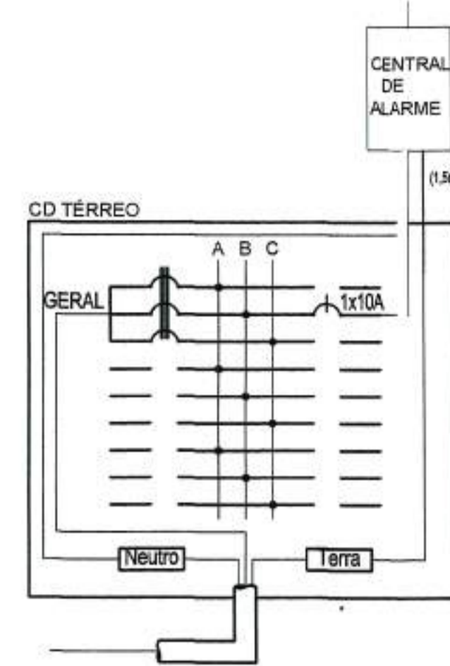
INSTALAÇÃO DA CENTRAL DE ALARME ESCALA 1:25
