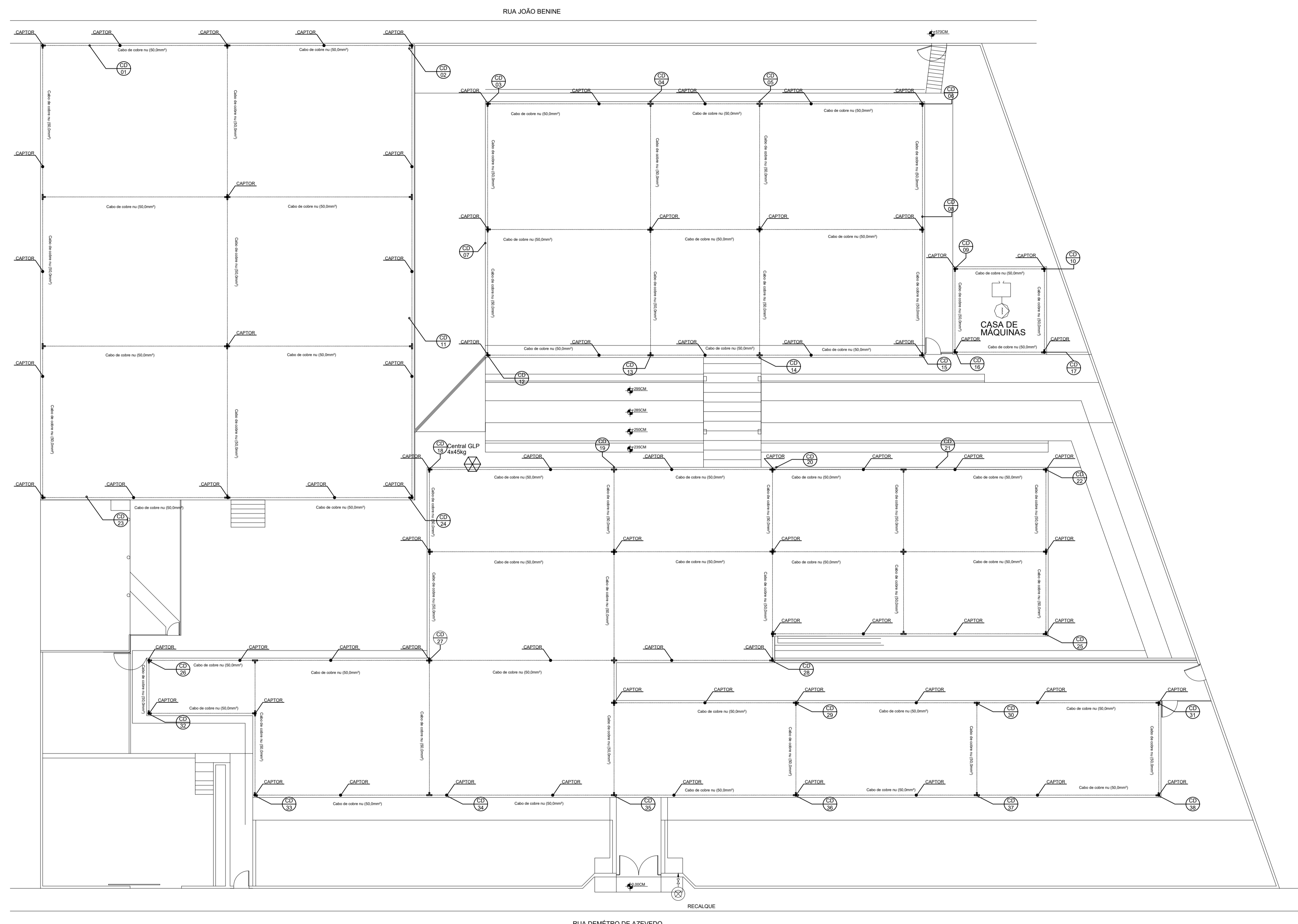
PLANTA BAIXA - CAPTORES / DESCIDAS Escala 1:125
