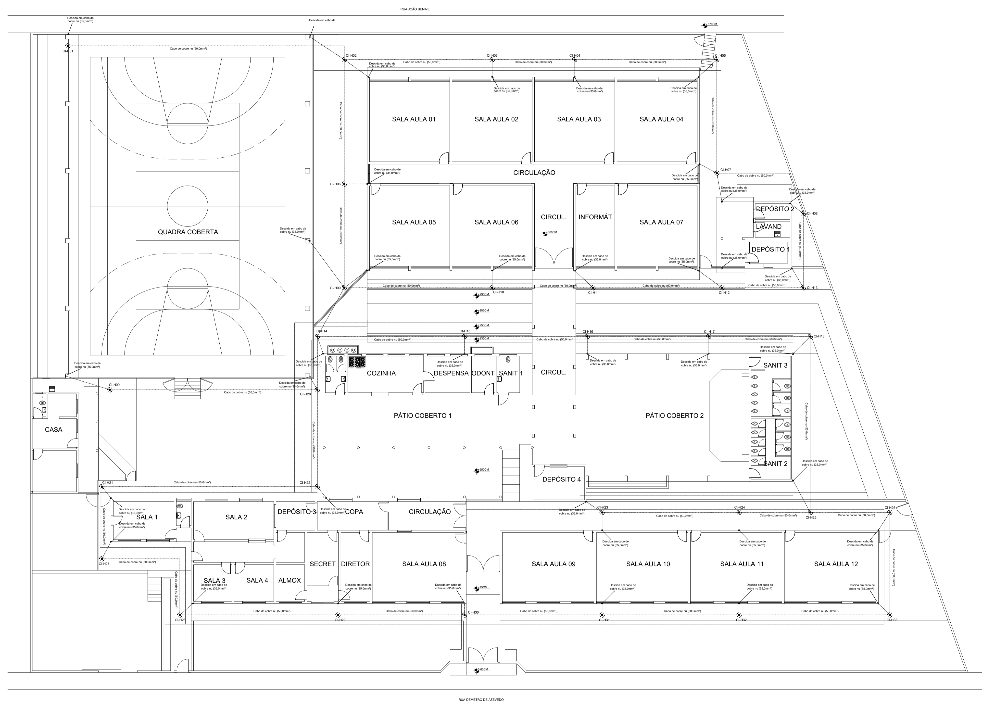
PLANTA BAIXA - MALHA DE ATERRAMENTO - CAIXA DE INSPEÇÃO/PASSAGEM Escala 1:125
