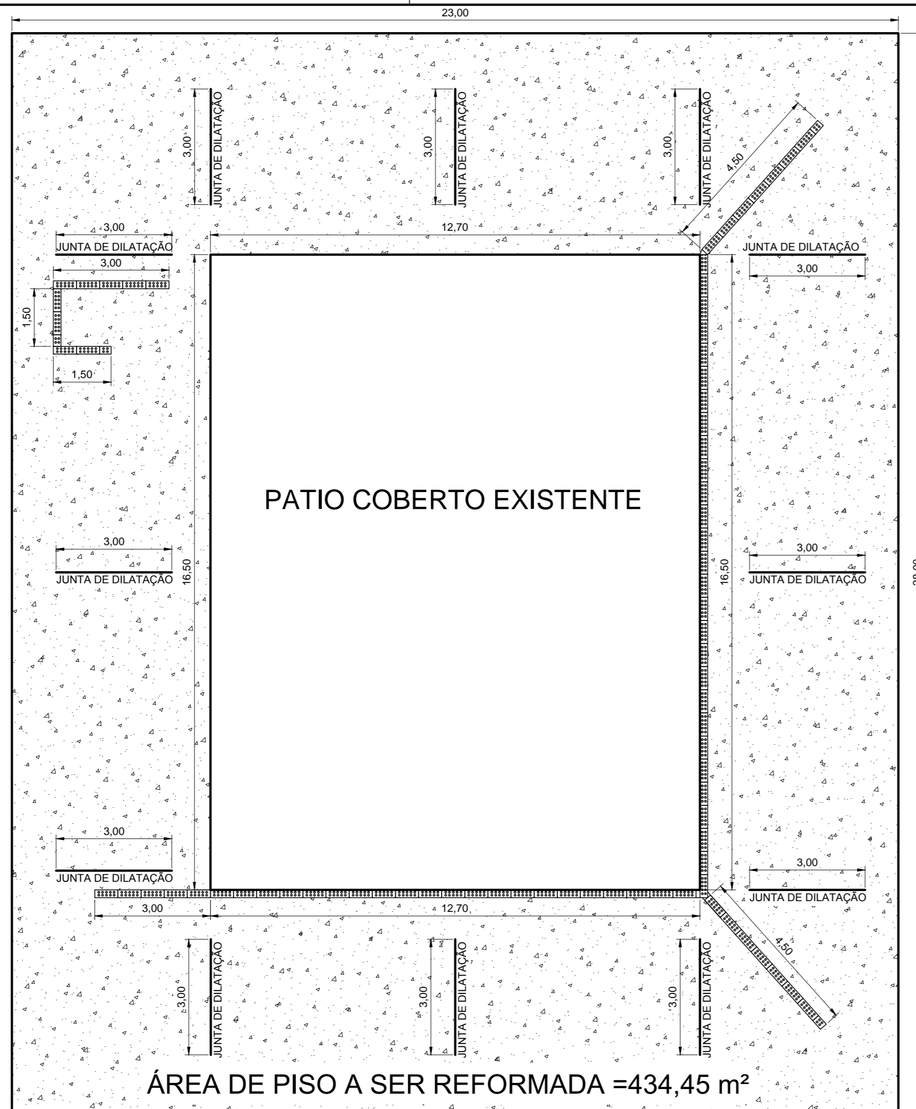
PLANTA BAIXA ESCALA: 1/100
